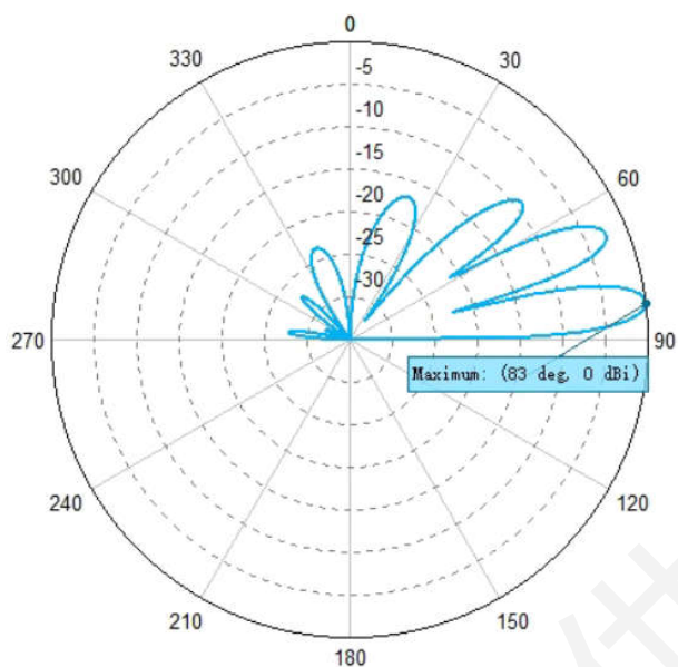
↑ 单天线 28.25MHz 方向图 (垂直面)
