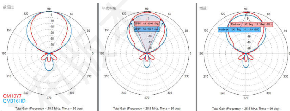
↑ 单天线 28.25MHz 方向图 (垂直面)
