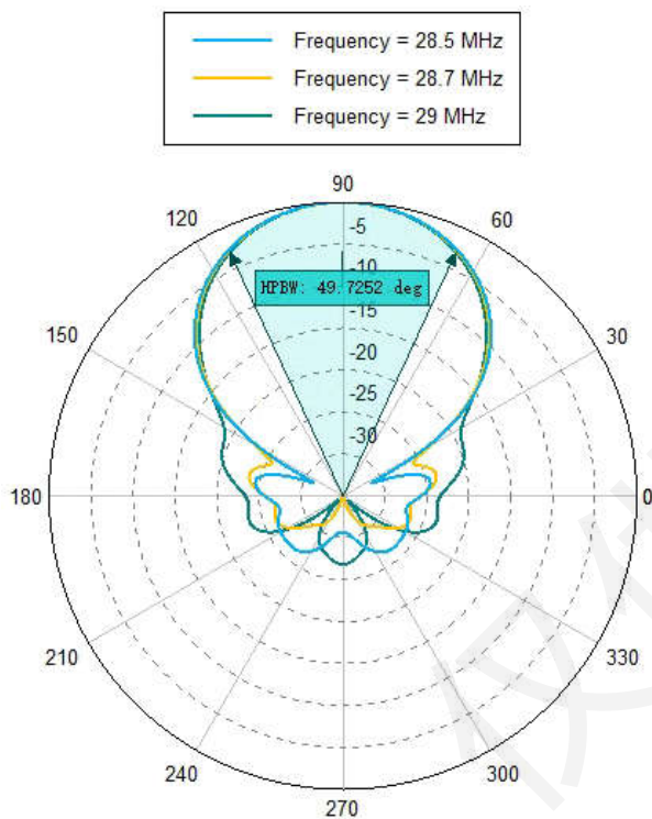
↑ 28.5~29MHz 方向图 (最大增益锥面)
