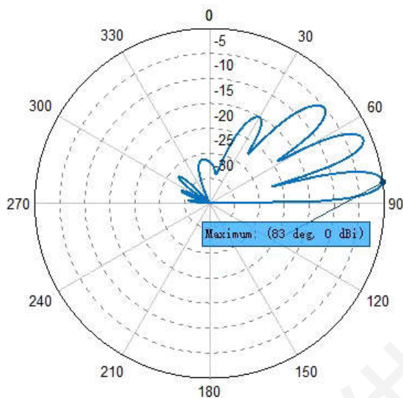
↑ 单天线 28.5MHz 方向图 (V 面, 高度 20 米)
