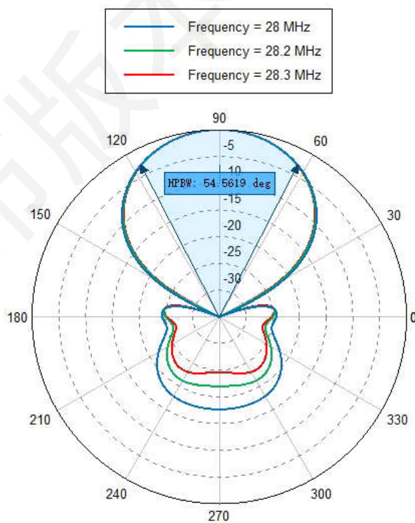
↑ 28MHz~28.5MHz 方向图 (最大增益锥面)
