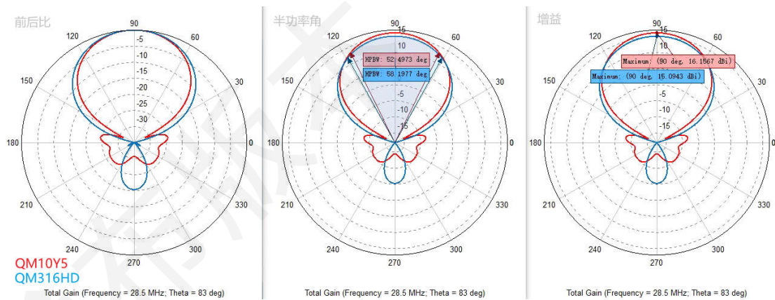
↑ 单天线 28.5MHz 方向图 (最大增益 H 面, 高度 20 米)
